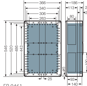
FP 0461 FP 0471
