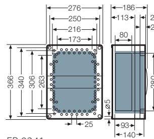
FP 0241 FP 0251
