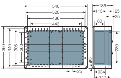
FP 0440 FP 0450
