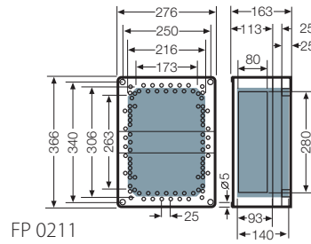
FP 0211 FP 0231
